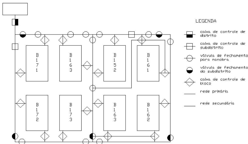
Subdivisão de rede em setores de medição e de manobra
