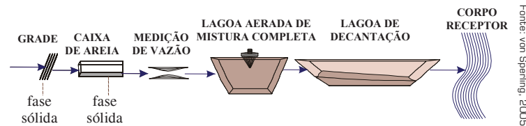
Lagoa aerada de mistura completa + lagoa de decantação
