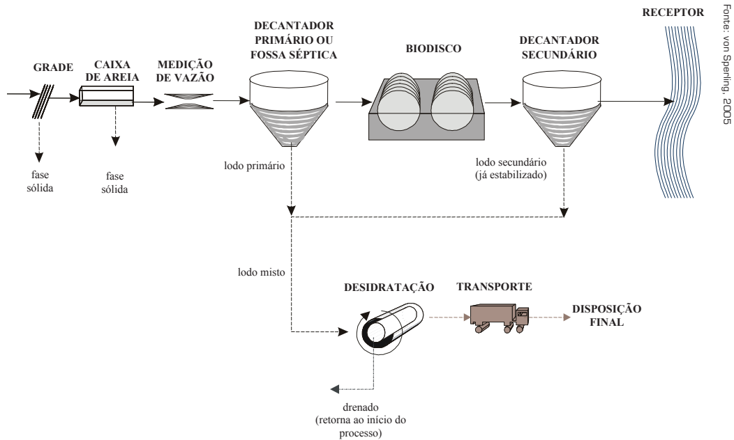
Biodiscos
